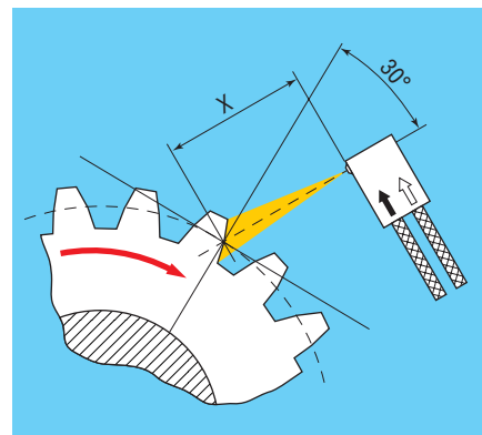
Принцип нанесения густой смазки на венцовую шестерню
